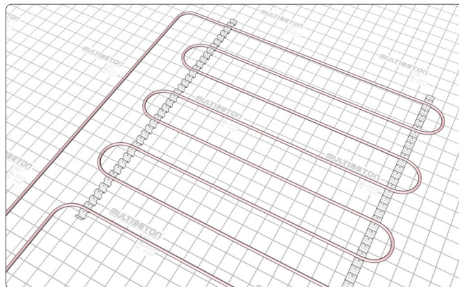
Verlegeart A25
