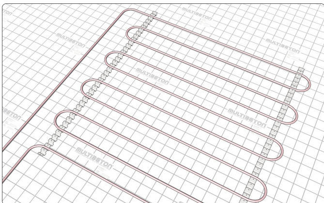
Verlegeart A20
